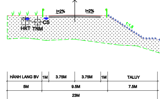
MẶT CẮT 2 -2 MẶT CẮT NGANG ĐỂ QUA KHU DẪN CỤ
