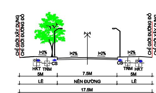
MẶT CẮT 3 - 3 MẶT CẮT NGANG ĐƯỜNG XÃ
