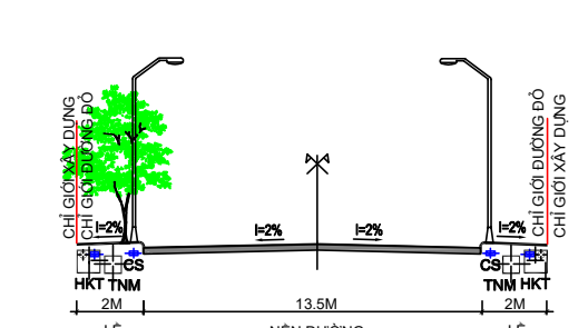
MẶT CẮT 5 - 5 MẶT CẮT NGANG ĐNĐ.0
