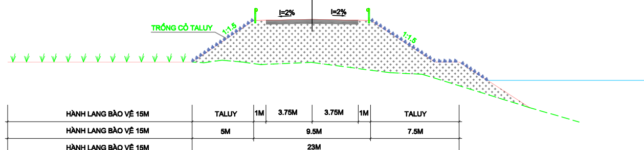
MẶT CẮT 2 -2 MẶT CẮT NGANG ĐỀ
