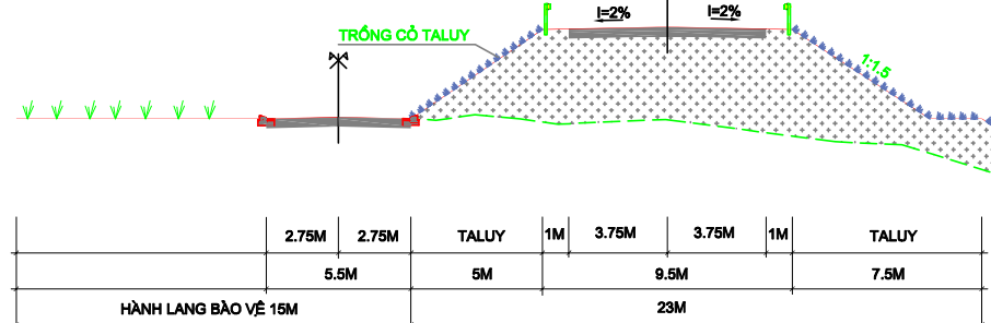
MẶT CẮT 2 -2 MẶT CẮT NGANG ĐỀ CÓ ĐƯỜNG LÊN ĐỀ
