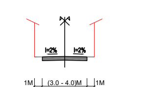
MẶT CẮT 6 - 6 MẶT
